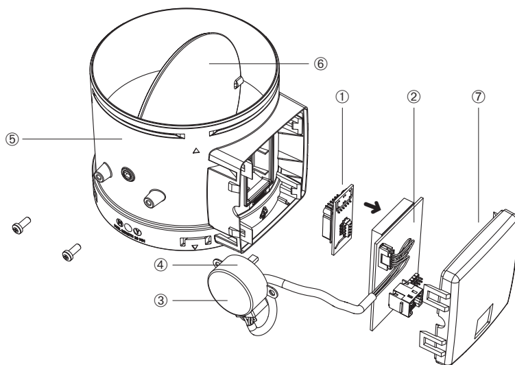
Regelmodule
