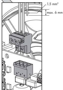
Aansluiten voedingskabel
