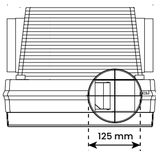
Bovenaanzicht
