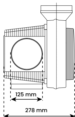
Zijaanzicht rechts
