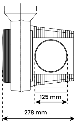
Zijaanzicht links
