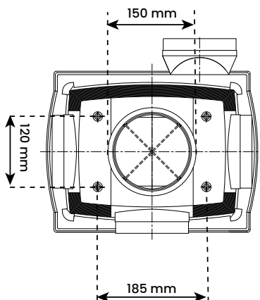
Achteraanzicht
